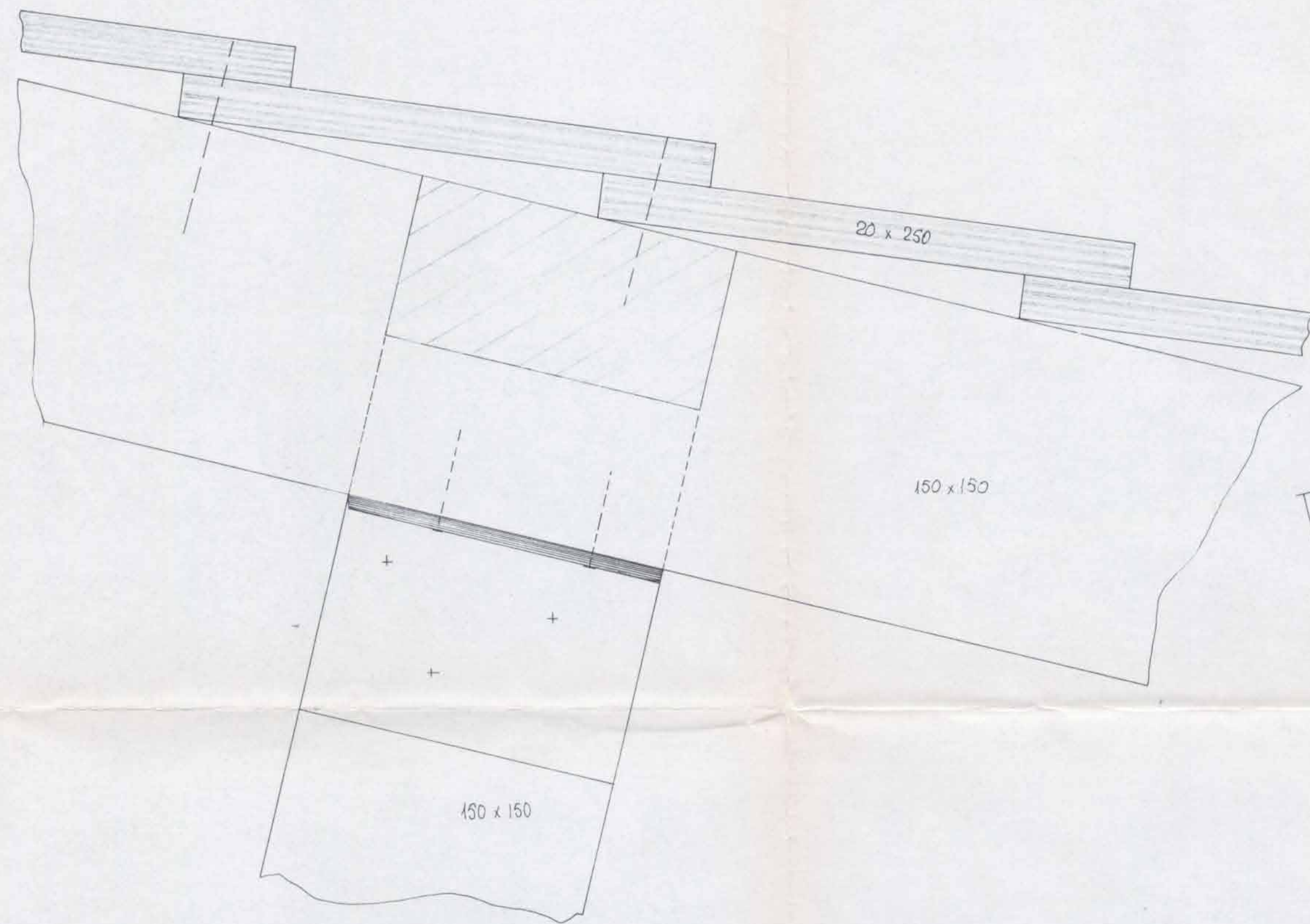
DETAIL DAKCONSTRUCTIE
