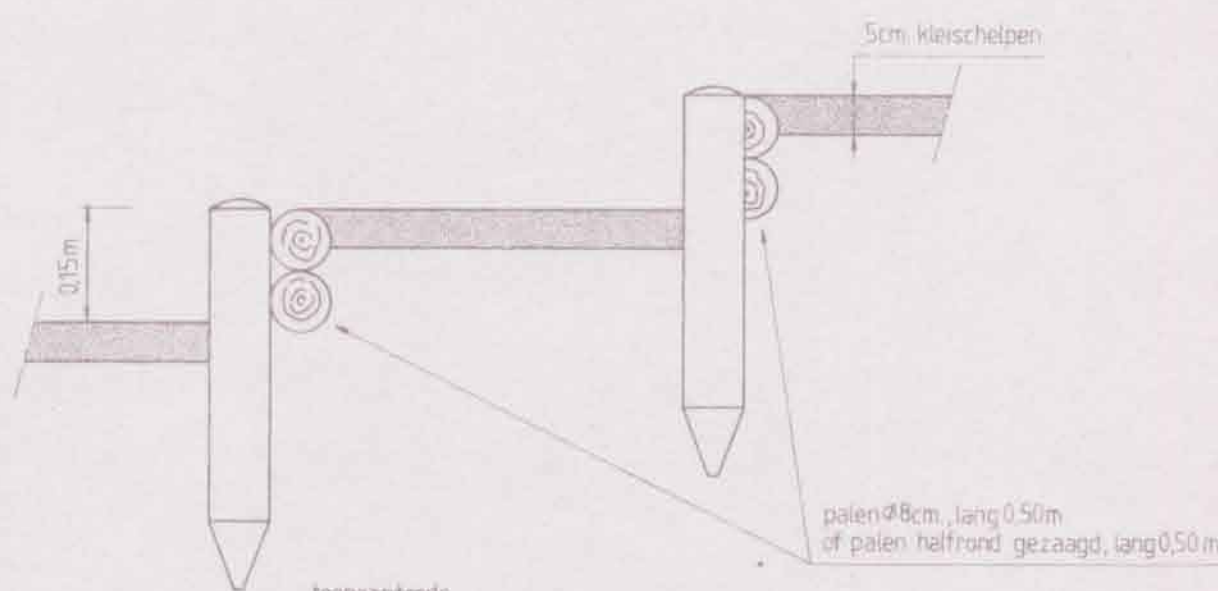
zijaanzicht luie trap schaal 1:10
