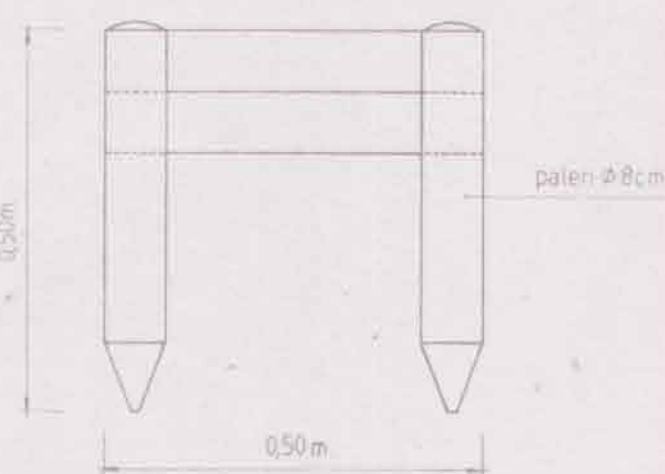
vooraanzicht luie trap schaal 1:10
