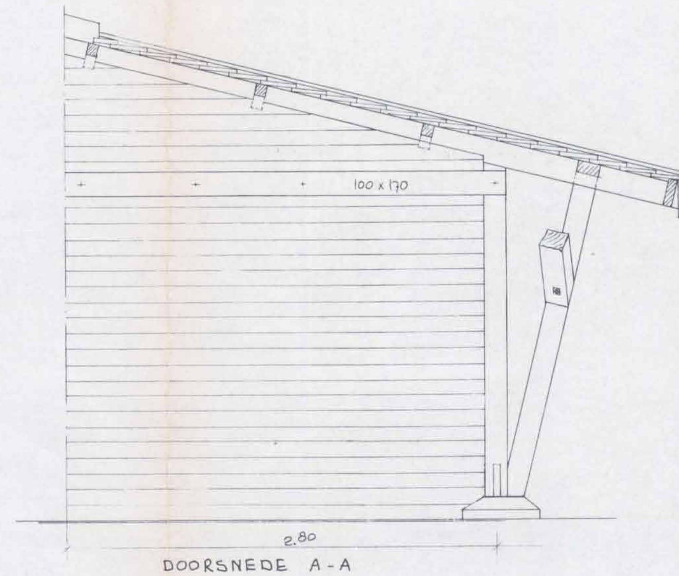
DOORSNEDE A-A
