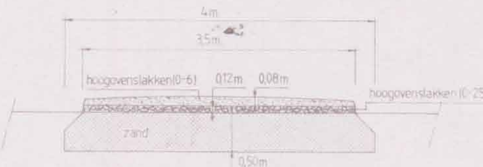
doorsnede B-B schaal 1:50
