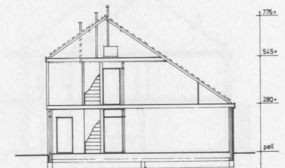
DOORSNEDE A-A
